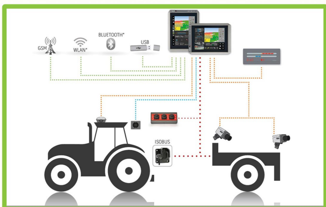
Isobus Vezérlés
